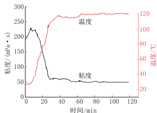
图5 120℃耐温耐剪切曲线
