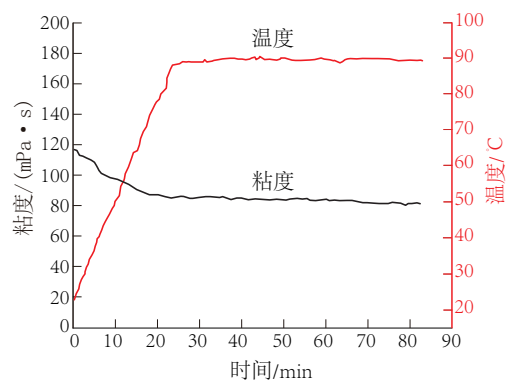
图4 90℃耐温耐剪切曲线
