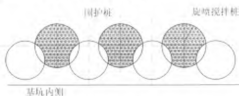
图2 围护结构示意图
