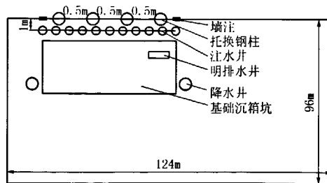
图1 冲床基础处理平面布置示意图
