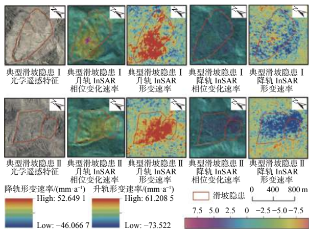
图5 典型滑坡隐患遥感特征图
