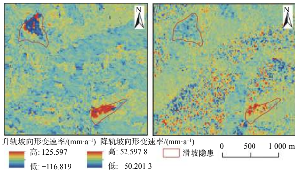
图9 后海村和水磨村滑坡隐患坡向形变图
