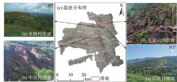
图6 隆德县滑坡隐患分布图
