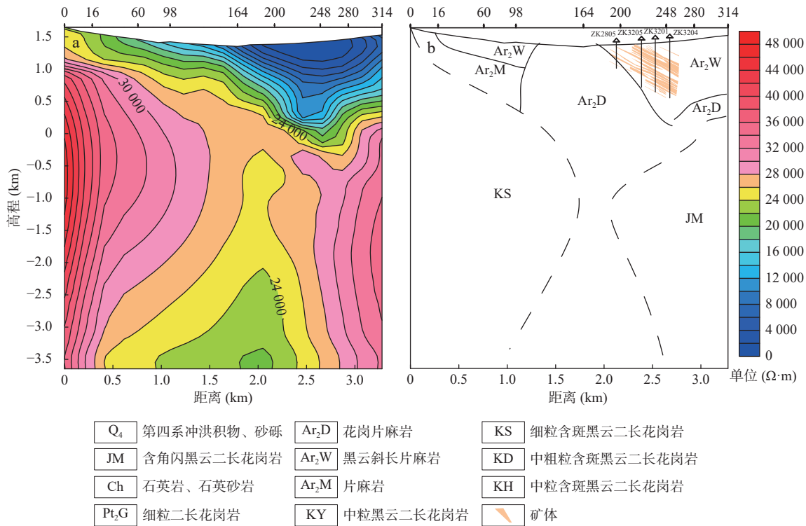
图4 Z2剖面MT电阻率反演剖面图(a)及地质解释图(b)
