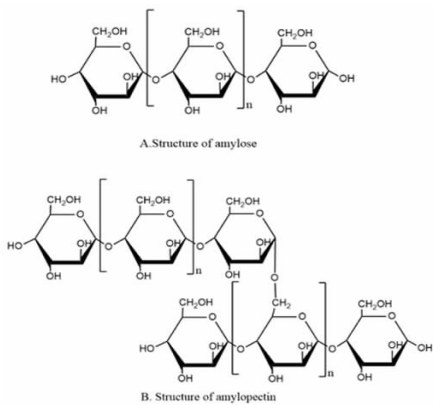
图 5 淀粉的结构
