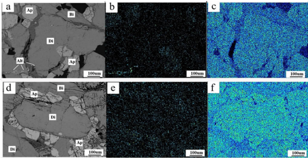
图 3 主要载钬矿物元素面扫描分布图 Fig. 3 Surface scanning distributions of scandium bearing minerals
