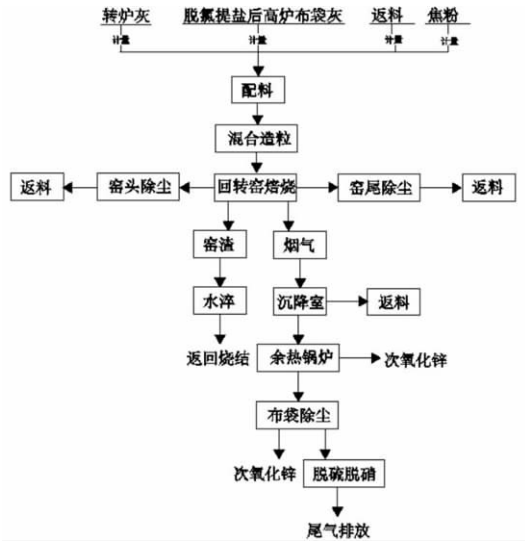
图 2 回转窑提锌工艺流程
