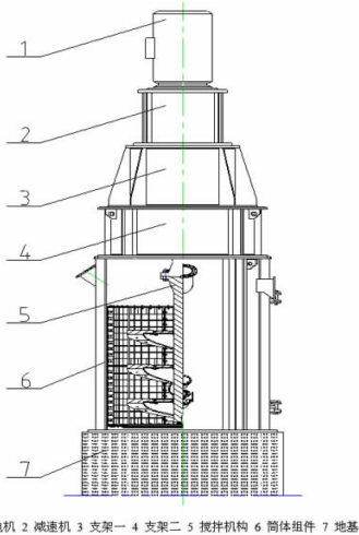
图 7 立式螺旋搅拌磨机结构简图 Fig. 7 Schematic diagram structure of vertical screw stirring mill
