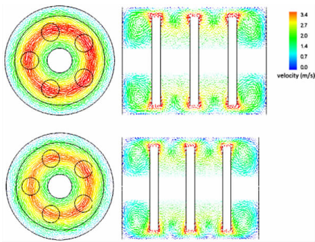
图3 搅拌细磨装备内矿浆运动状态分布情况
