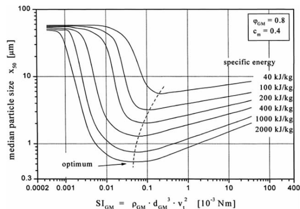
图2 产品粒度与应力强度以及输入能量的关系
