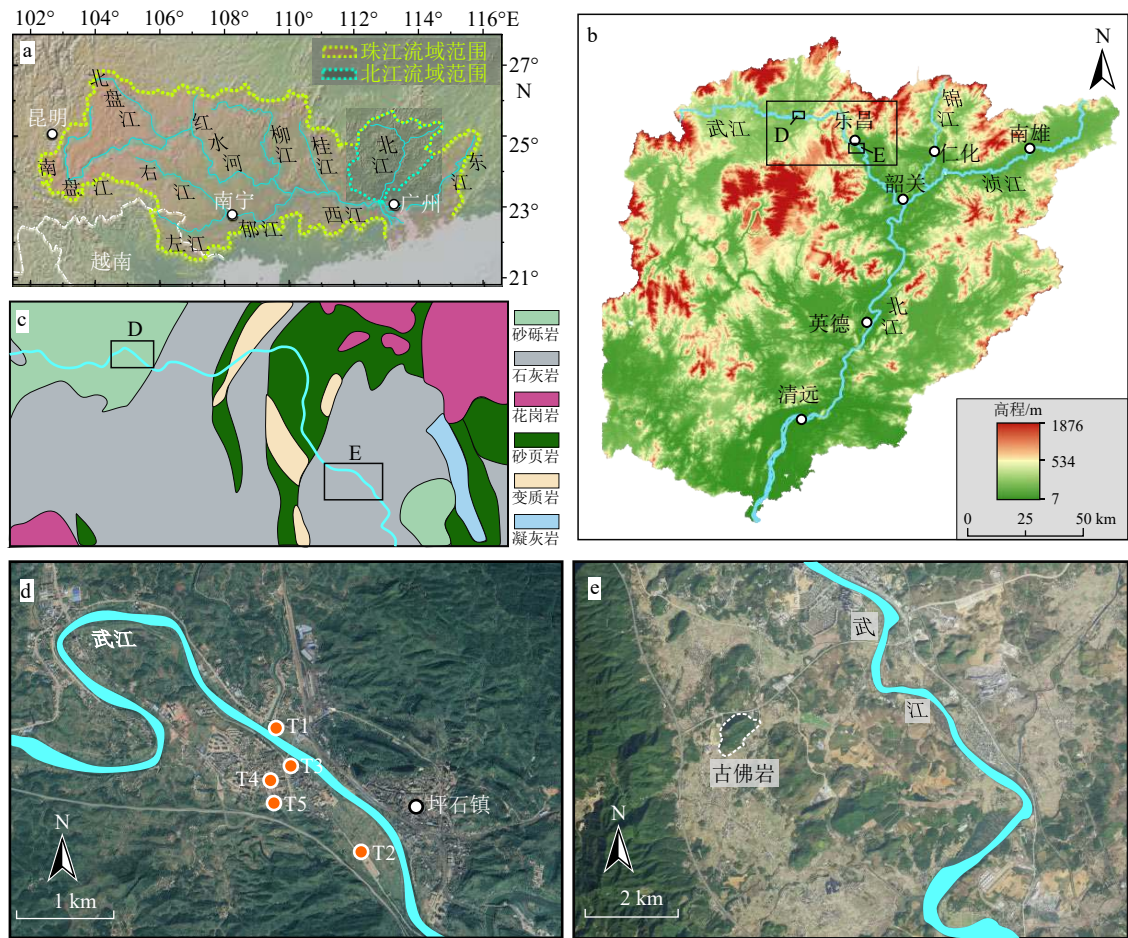
图 1 北江上游坪石盆地河流阶地和古佛岩地理位置
