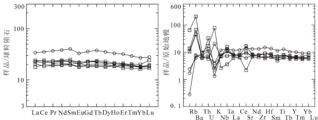
图6 东沟蛇绿岩的基性火山岩球粒陨石标准化稀土元素分配模式和原始地幔 标准化微量元素蛛网图(标准化数据均引自参考文献[19])
