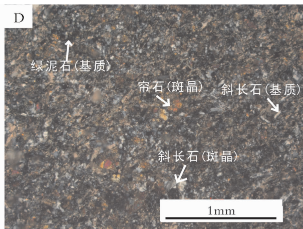
绿泥石化细碧岩显微特征(5×10,+)
