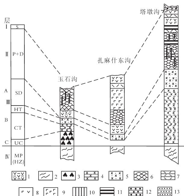
图 8 北祁连山大洋扩张脊与弧后扩张脊蛇绿岩柱状序列对比图
