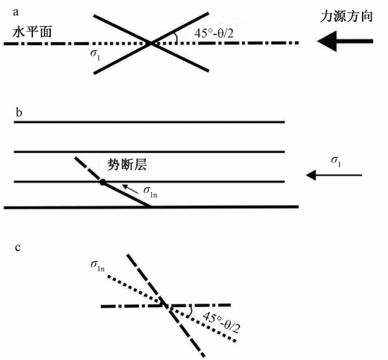
\theta —岩石内摩擦角； \sigma_1 —区域挤压应力； \sigma_{1n} —先存断层活动引起的主压应力 a—安德森断裂模式；b—先存断层复活；c—二次断裂倾角
