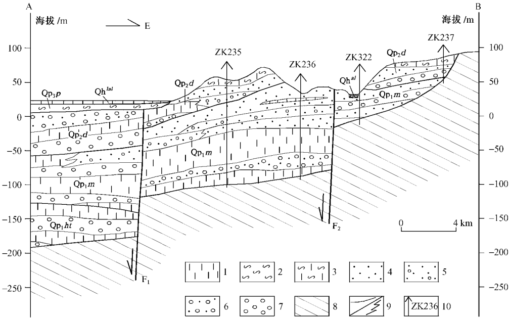
图 3 阳罗—黄沙街第四纪地质剖面（剖面位置见图 2 中 A—B 剖面线）
