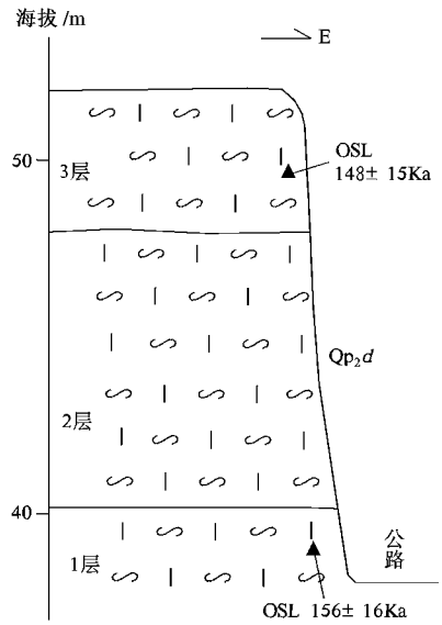
图 4 荣家湾露头剖面 Fig.4 Rongjiawan outcrop section 分层岩性详见正文说明，OSL-光释光测年
