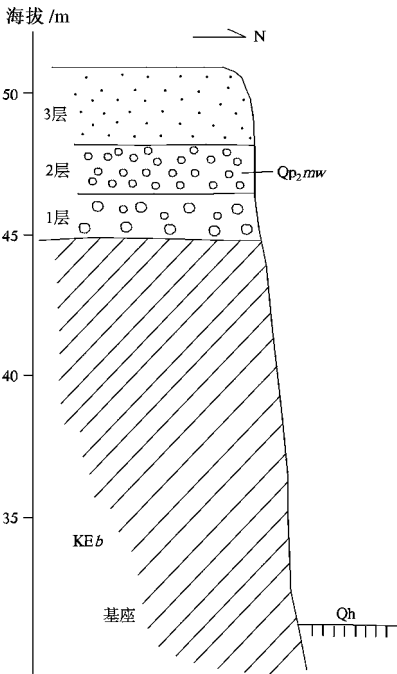
图 6 傅家垸第四纪地质露头剖面
