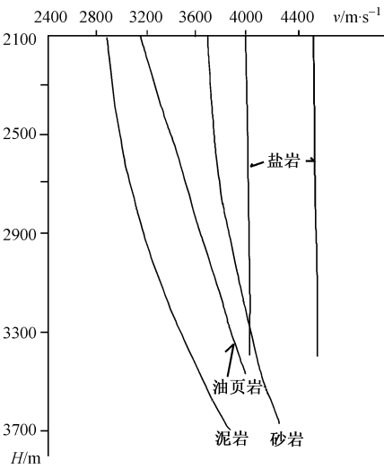
图2 文留油田不同岩性速度-深度变化特征
